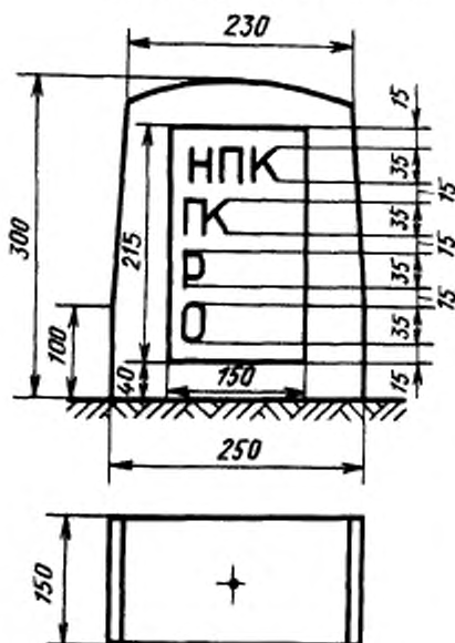
Начало переходной кривой
