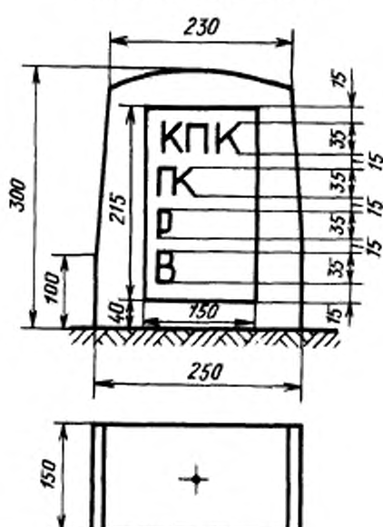
Конец переходной кривой
