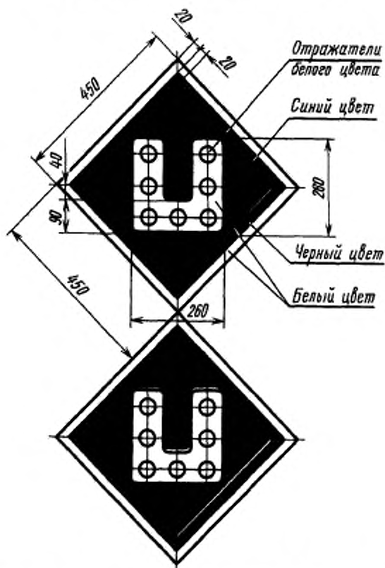
Знак «ВКЛЮЧИТЬ ТОК НА ЭЛЕКТРОПОЕЗДЕ»
