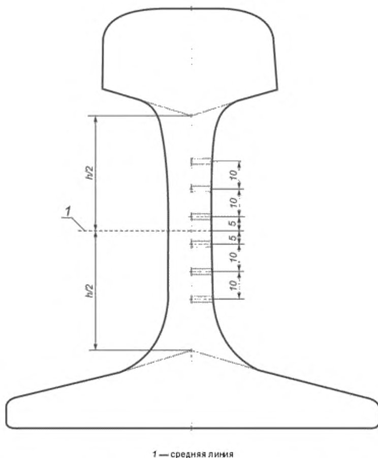
Рисунок К.4 — Расположение отражателей в шейке образца
