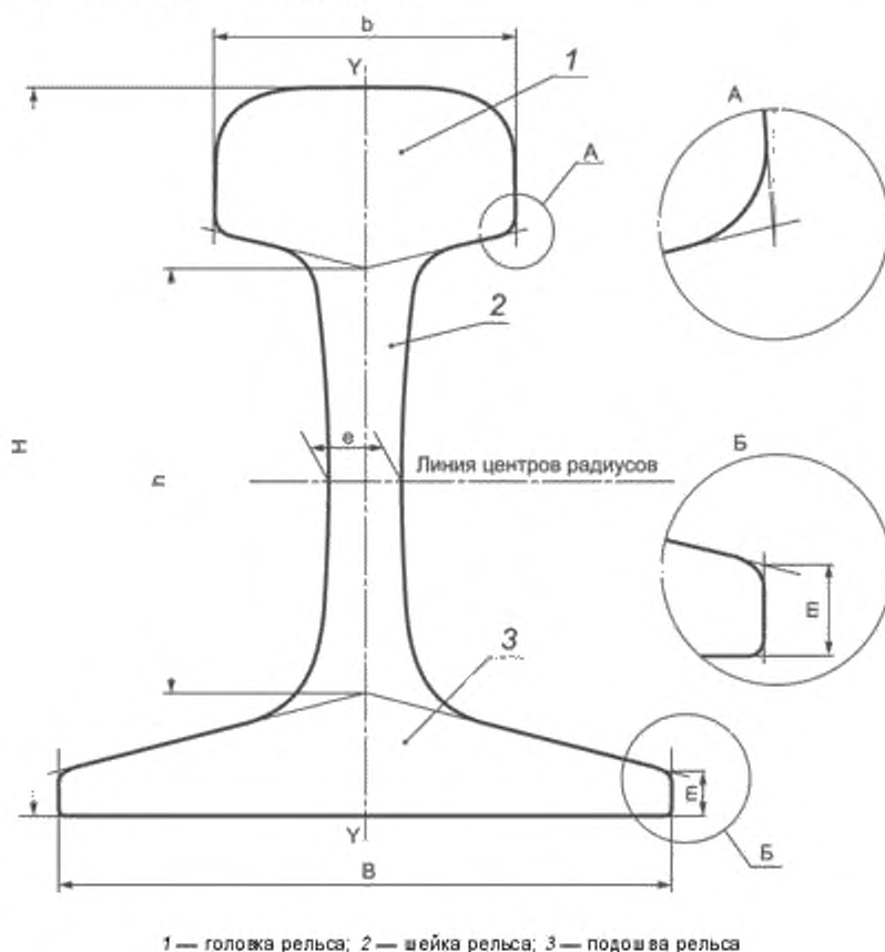
Рисунок 1 — Основные размеры поперечного сечения рельса
