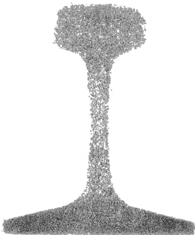
Рисунок И.1 — Макроструктура без ликвации (серный отпечаток)
