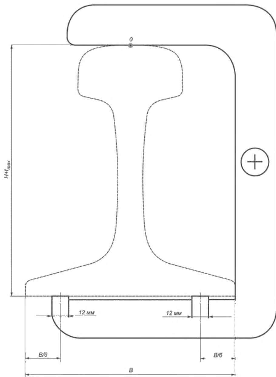
Рисунок ЖЗ — Шаблоны контроля высоты рельса
