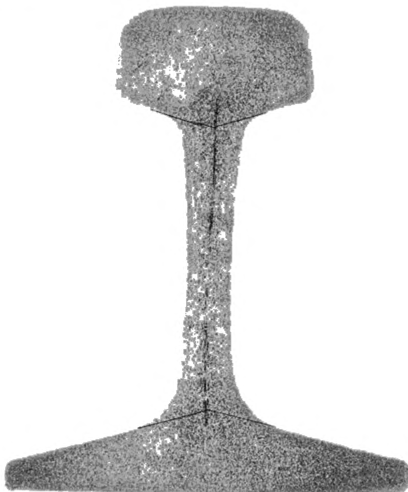
Рисунок И.5 — Осевая ликвация в шейке, простирающаяся в головку и (или) в подшву (серый отпечаток)
