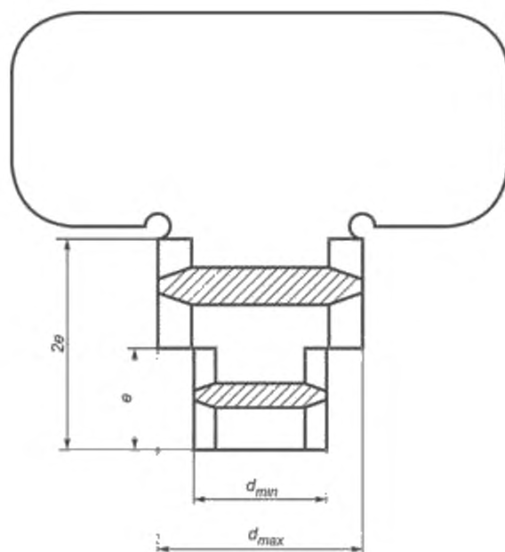
Рисунок Ж13 — Шаблон контроля диаметра болтовых отверстий
