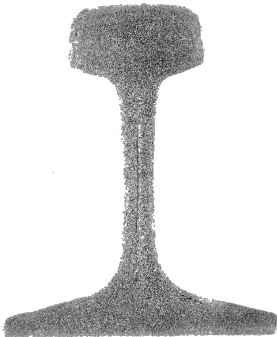
Рисунок И.13 — Ликвационные полосы (серый отпечаток)
