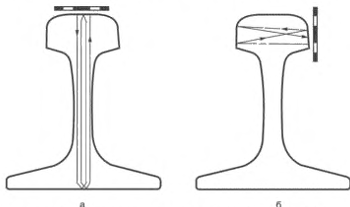
Рисунок К.1 — Схемы сканирования при НК рельсов методом А
