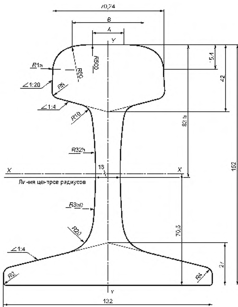
Рисунок Г.1 — Рельс типа Р50
