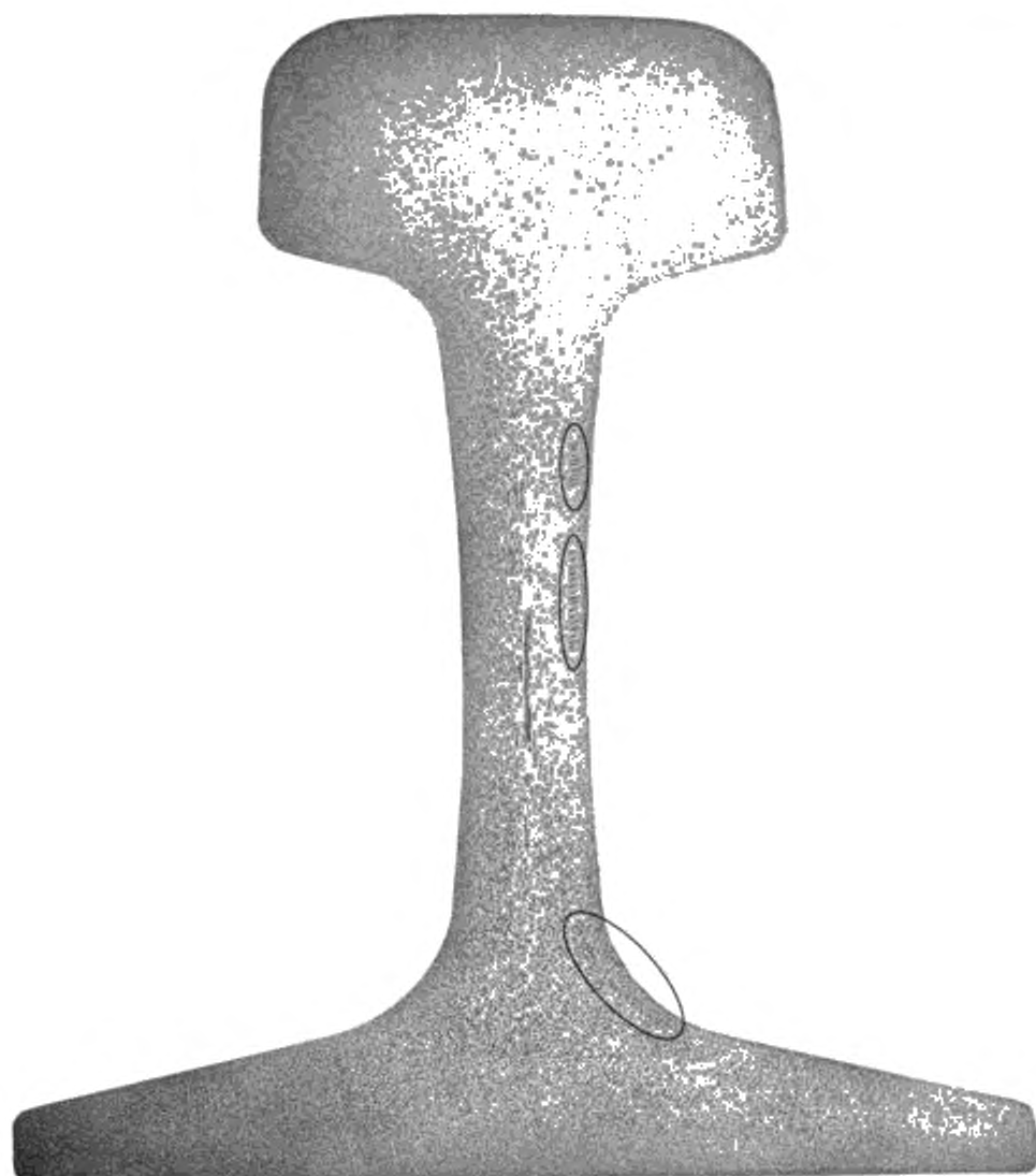
Рисунок И.16 — Группа ликвационных полосок с общей протяженностью более 20 мм при протяженности каждой полоски менее 3 мм (глубокое травление)
