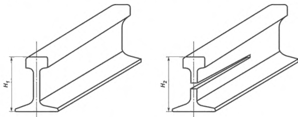
Рисунок 5 — Схема определения остаточных напряжений в шейке рельсов
