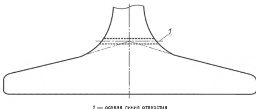
Рисунок К.5 — Расположение отражателя в подшве образца
