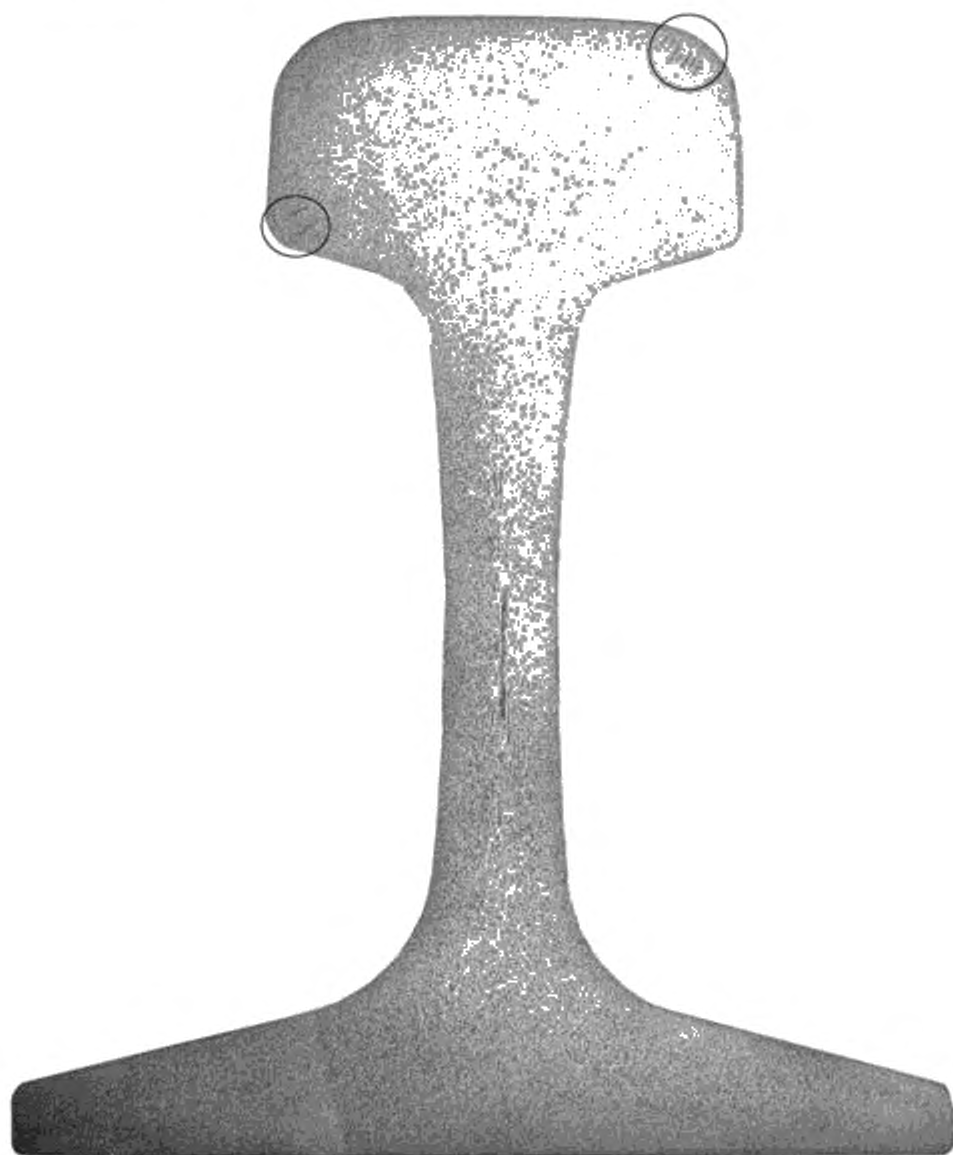
Рисунок И.15 — Группа ликвационных полосок с общей протяженностью более 6 мм при протяженности одной полоски более 3 мм (глубокое травление)
