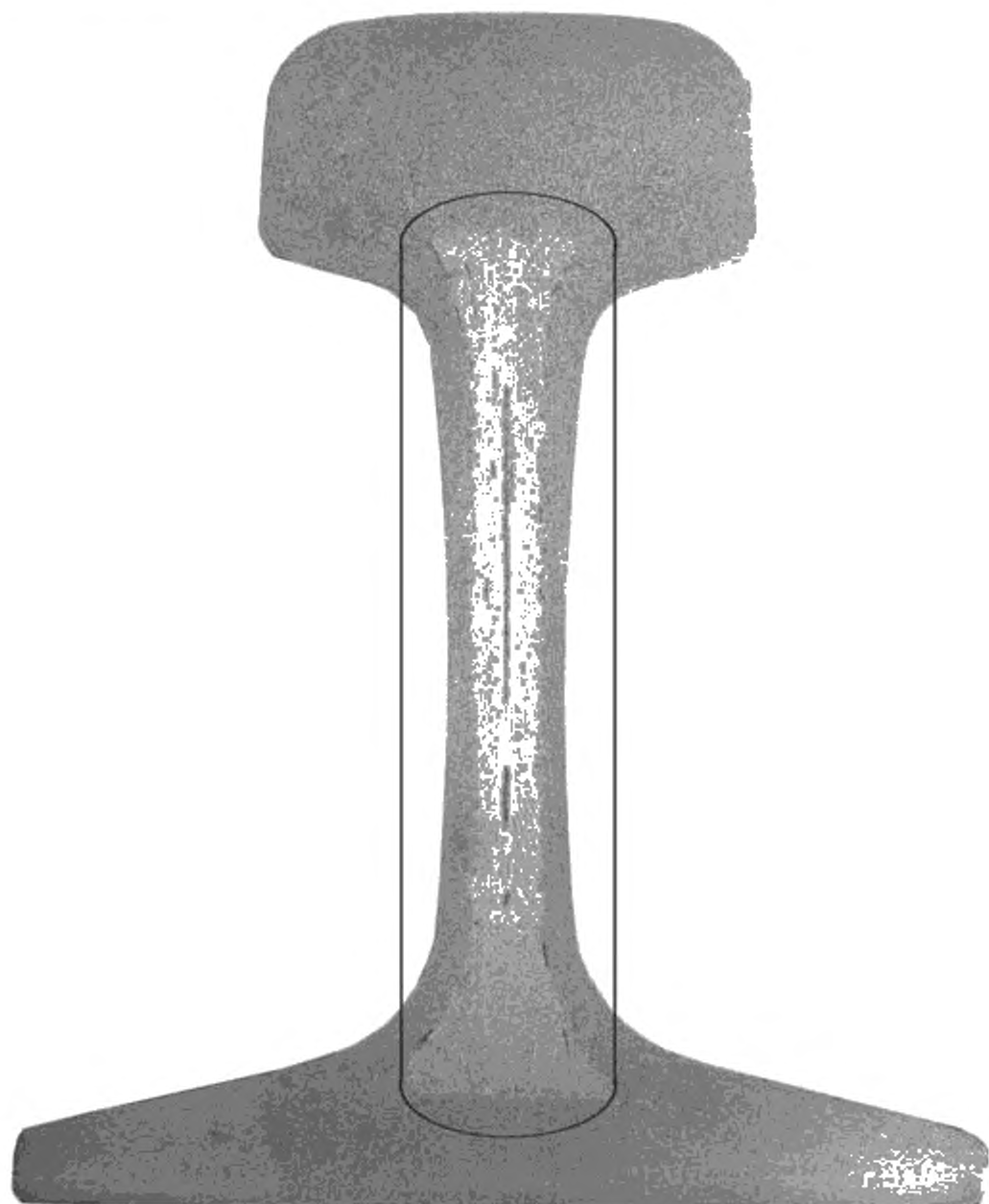
Рисунок И.7 — Ликвационная зона, имеющая ширину, превышающую 1/3 толщины шейки (глубокое травление)
