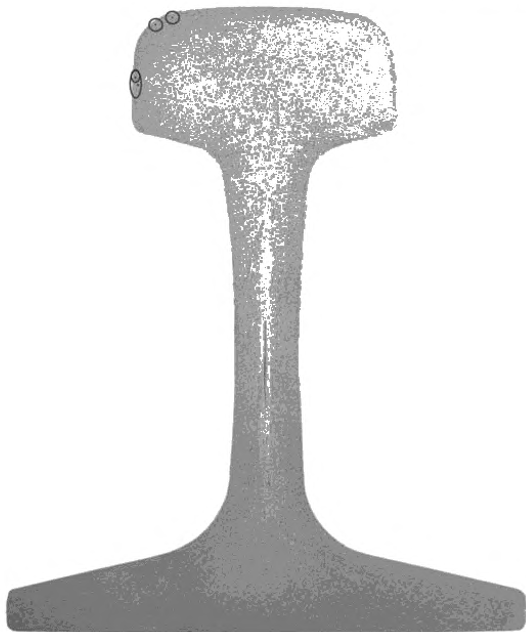
Рисунок И.10 — Наличие более 3 одиночных точек в одном элементе профиля (глубокое травление)
