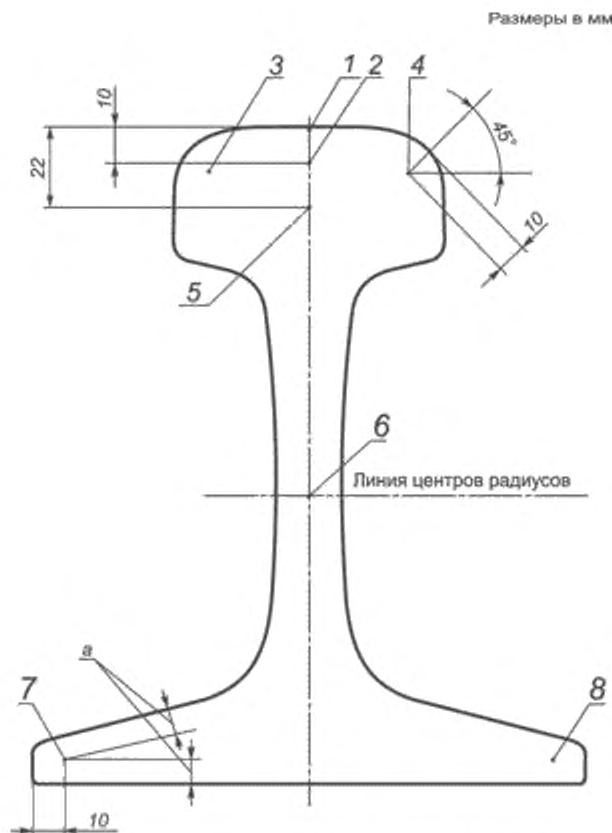
Рисунок 3 — Точки измерения твердости рельсов
