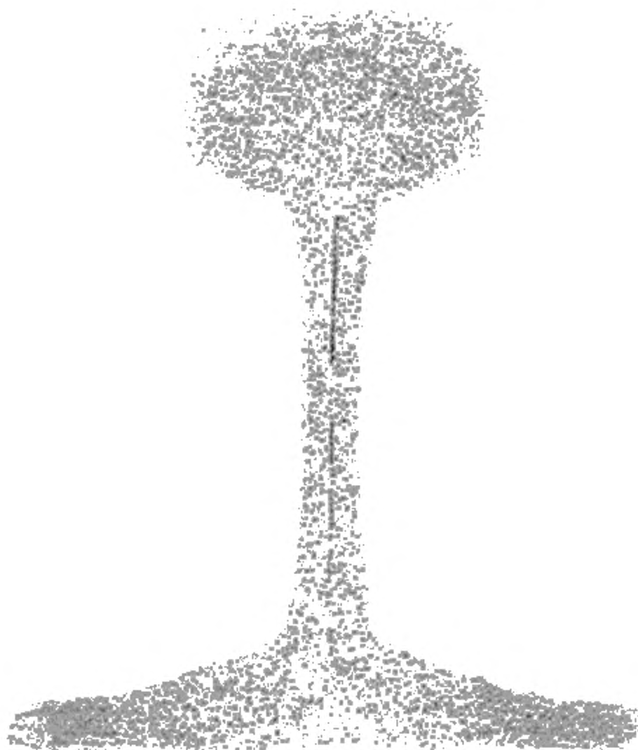
Рисунок И.4 — Незначительная прямая ликвация (серый отпечаток)
