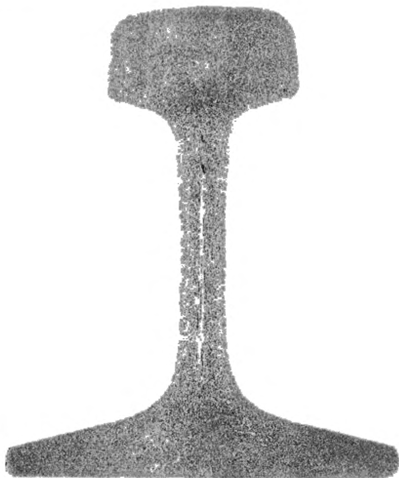
Рисунок И.3 — Обратная ликвация в шейке (серый отпечаток)
