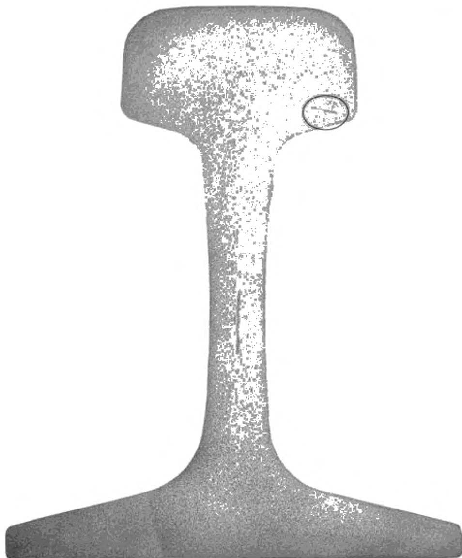
Рисунок И.14 — Одиночные ликвационные полосы с длиной более 5 мм (глубокое травление)
