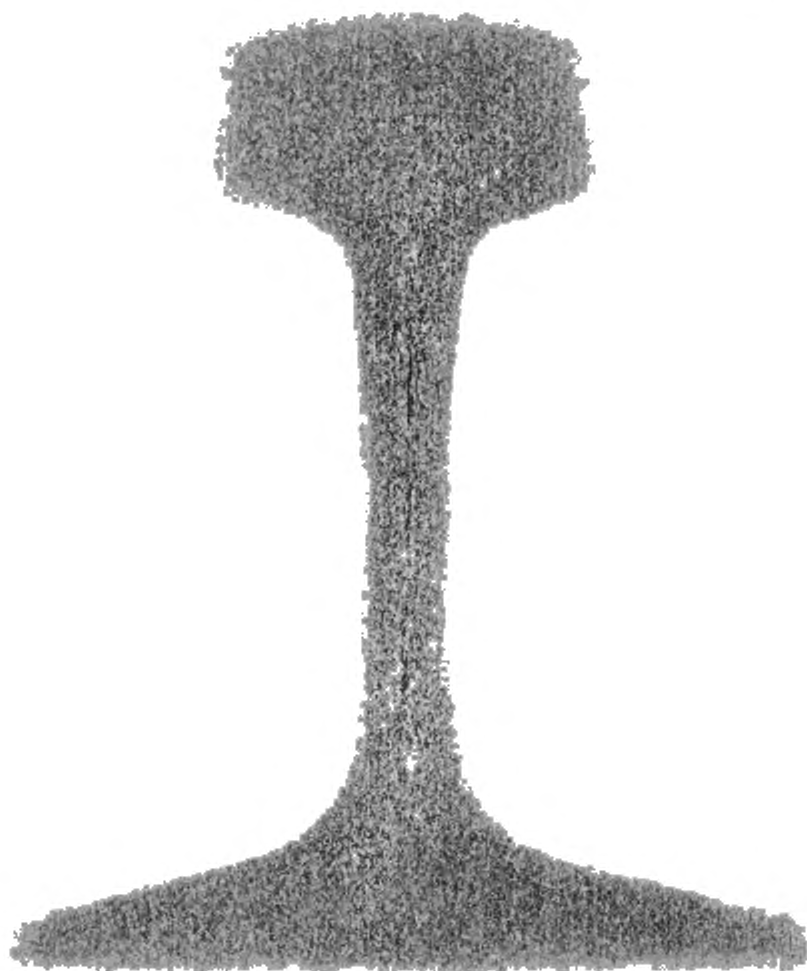
Рисунок И.4 — Незначительная прямая ликвация (серный отпечаток)
