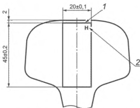
Надрез наносят со стороны верха образца (стрелка 1), верх образца обозначают клеймом «Н» на торце образца (стрелка 2)
