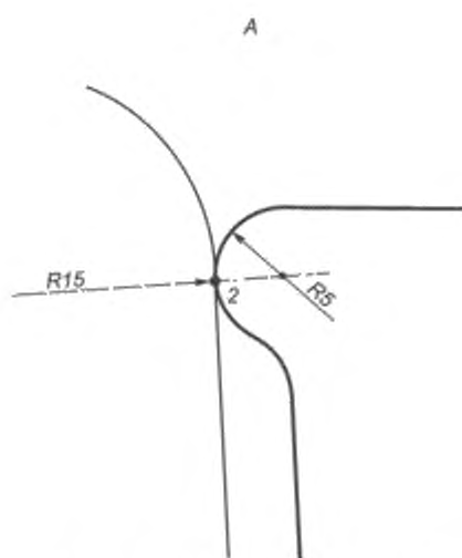
Рисунок Ж.6 — Шаблоны контроля несимметричности рельса
