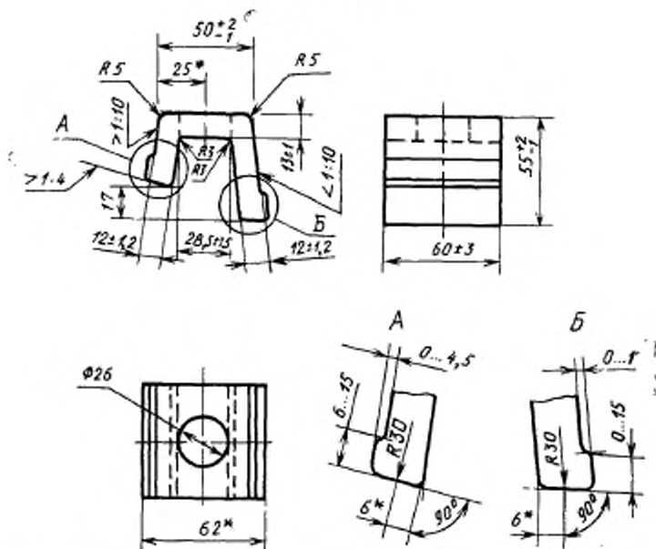
Клемма ПК
